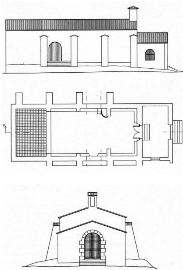
Fig. 15: Planta i alçats de l'Ermite de Santa Bàrbara de Cocentaina. Font: Domènech 2003.
