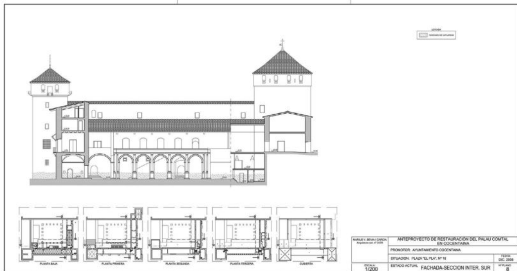
Fig. 10: Plantes i secció de les diferents altures del Palau Comtal de Cocentaina (Cortesia: Màrius Bevià).
