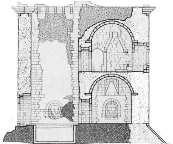
Fig. 8: Secció de la Torre Gòtica del Castell de Cocentaina abans de la seua restauració. Font: Portela 2003.
