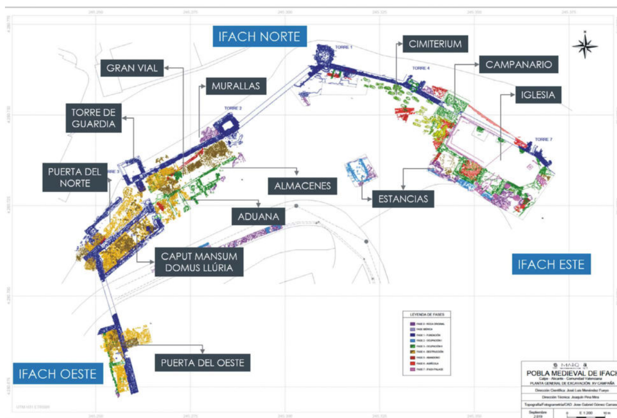
Fig. 1: Planta de les restes excavades de la Poble d'Ifac a Calp. La duana i els magatzems són les zones d'ampliació de les obres de na Margarida, a partir de l'any 1325. ADT MARQ.
