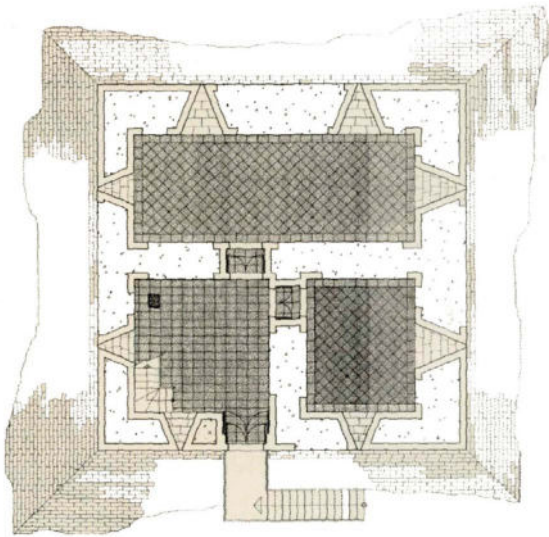
Fig. 7: Planta de la Torre Gòtica del Castell de Cocentaina abans de la seua restauració. Font: Portela 2003.
